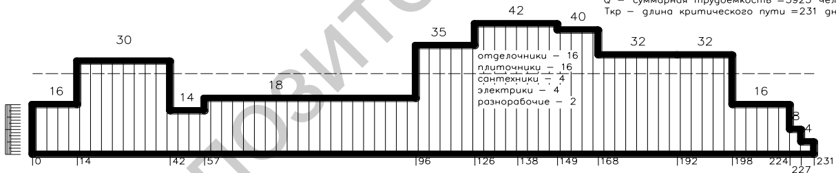
График потребности в трудовых ресурсах (в сутки)
